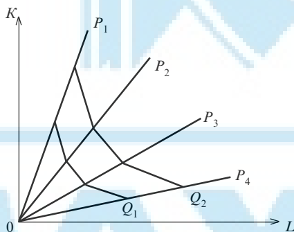
Рис. 12. Ломаная изокванта
