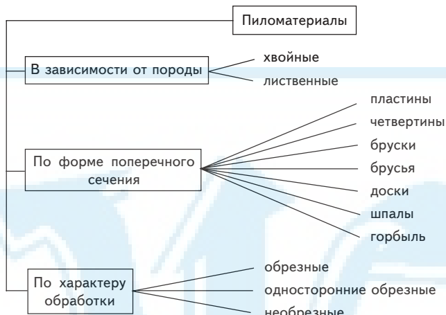
Рис. 12.3. Классификация пиломатериалов
