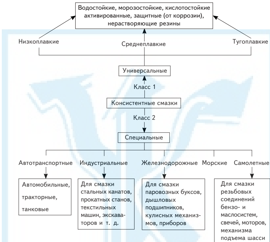
Рис. 6.3. Классификация консистентных смазок
