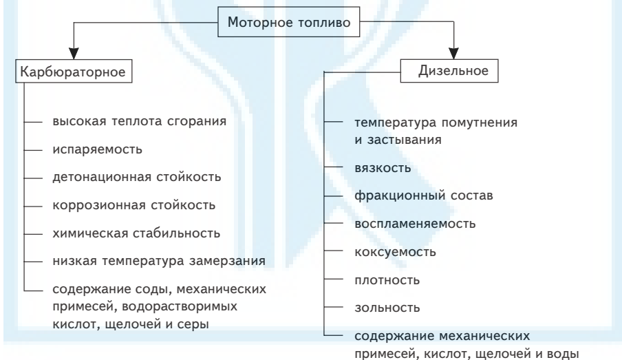
Рис. 5.4. Требования, предъявляемые к моторным топливам и их характеристики
