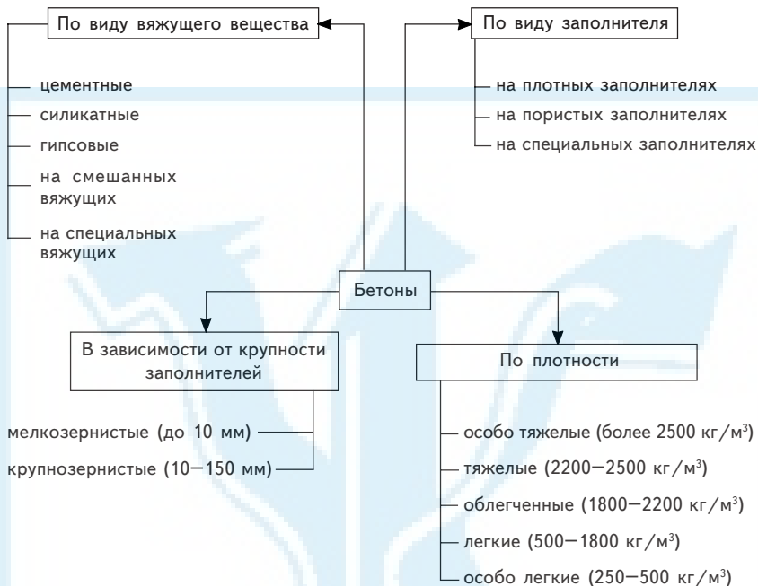
Рис. 11.3. Классификация бетонов
