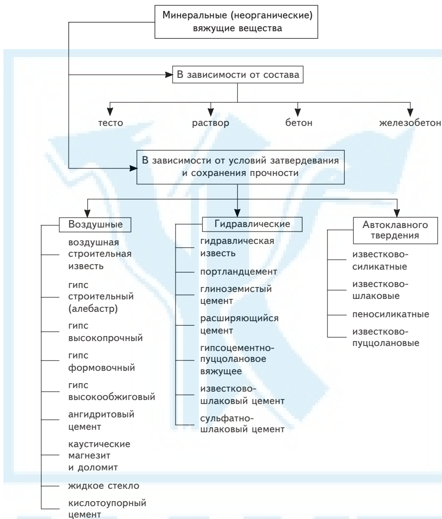
Рис. 11.1. Классификация минеральных вяжущих веществ
