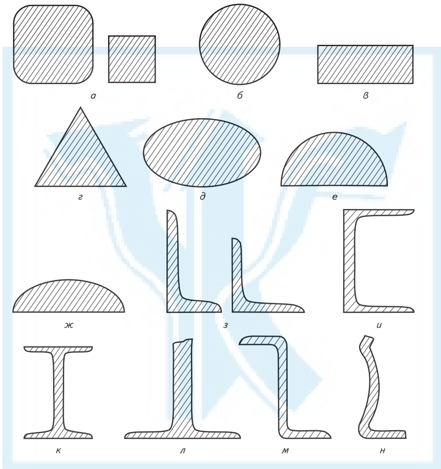
Рис. 2.4. Основные виды сортового проката:
