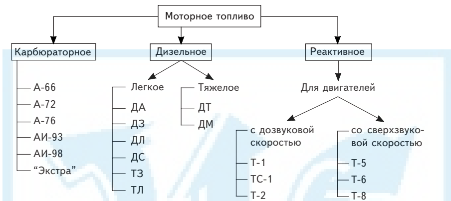
Рис. 5.3. Виды и марки моторных топлив
