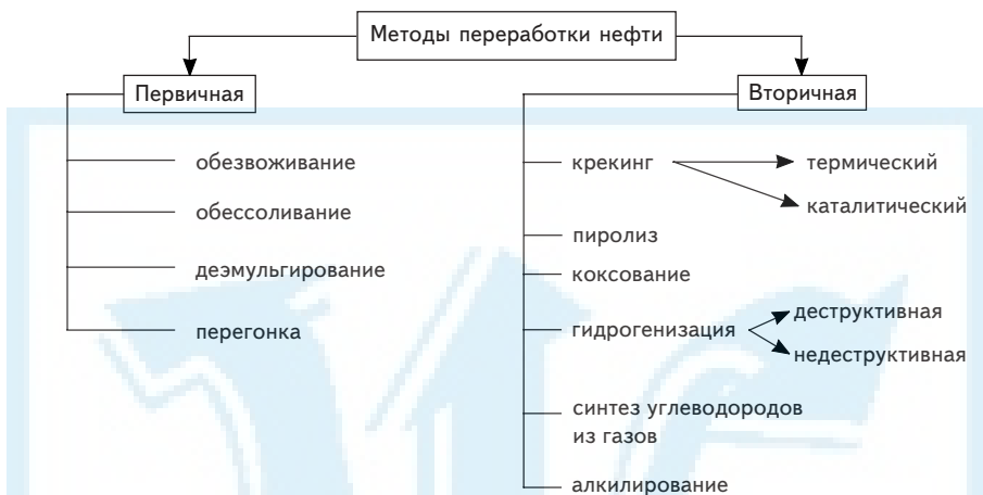
Рис. 5.2. Методы переработки нефти
