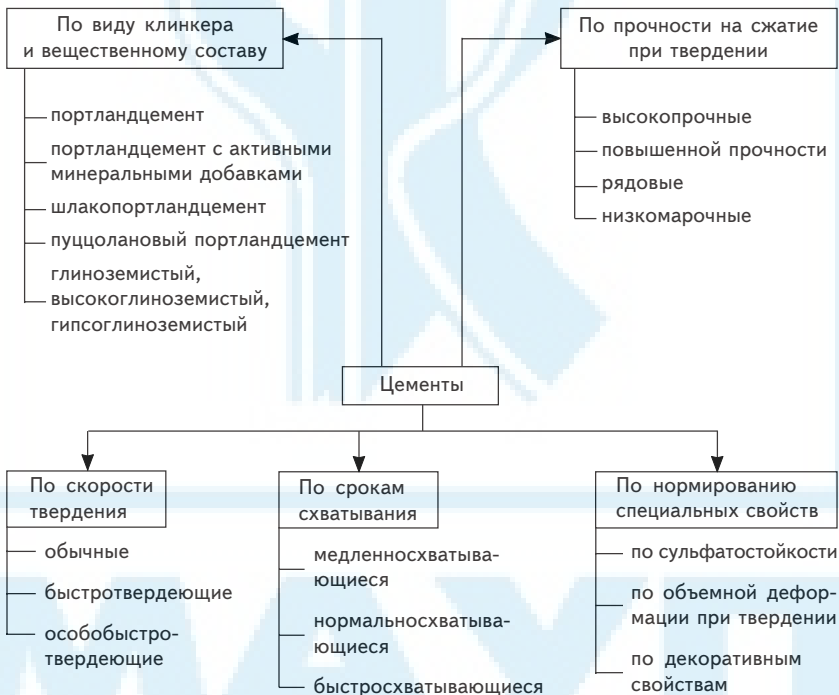
Рис. 11.2. Классификация цементов
