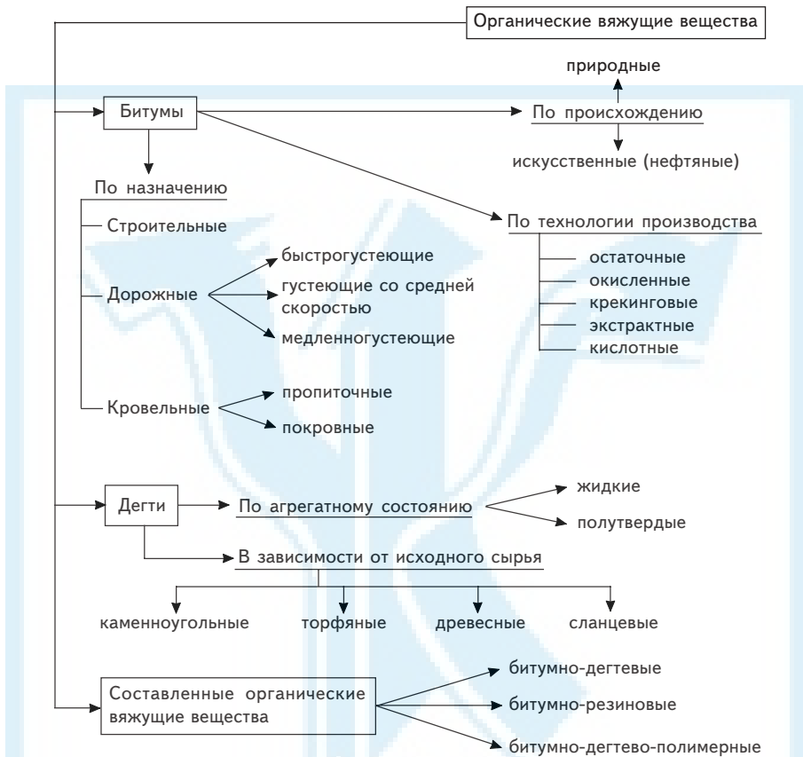
Рис. 11.4. Классификация органических вяжущих веществ
