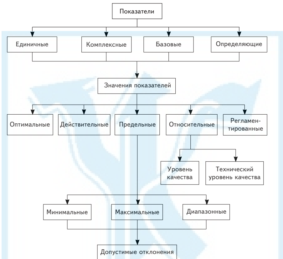
Рис. 1.3. Классификация показателей качества
