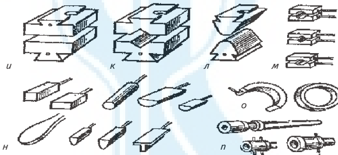
Рис. 3.5. Виды кузнечного инструмента для ручной и машиннойковки:
