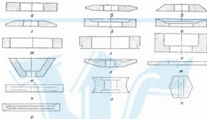
Рис. 3.2. Виды шлифовальных кругов:
